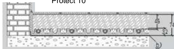
2. Speciel lav konstruktion Protect 10
