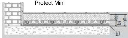
7. Lav konstruktion i nyt eller renoverede byggeri Protect Mini
