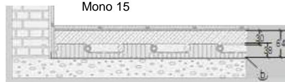
6. Speciel lav konstruktion Mono 15
