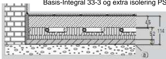
5. Konstruktion mod jord eller uopvarmede rum Basis-Integral 33-3 og extra isolering PS 20
